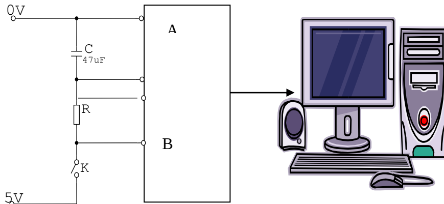
Hình 4. Sơ đồ mạch thí nghiệm về sự nạp điện của tụ điện
