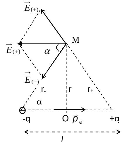
Hình 7- 6 Điện trường gây bởi lưỡng cực điện
