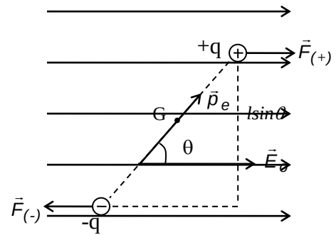
Hình 7 - 8. Lưỡng cực điện trong điện trường đều
