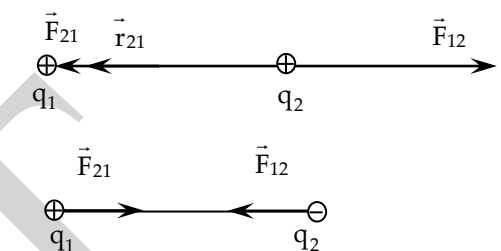
Hình 7-2 Lực tương tác giữa hai điện tích điểm.
