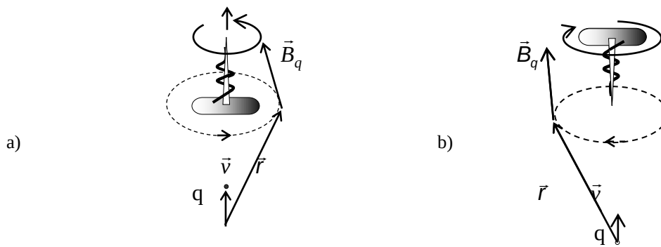
Hình 10-10. Vectơ cảm ứng từ \vec{B}_q do điện tích q chuyển động gây ra. a) q > 0 , b) q < 0
