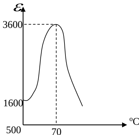
Hình 9-5a Sự phụ thuộc của \epsilon vào nhiệt độ
