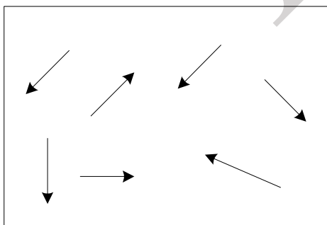
Hình 12-6a: ( B_0 = 0 )
