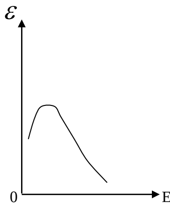
Hình 9-5b Sự phụ thuộc của \epsilon vào E
