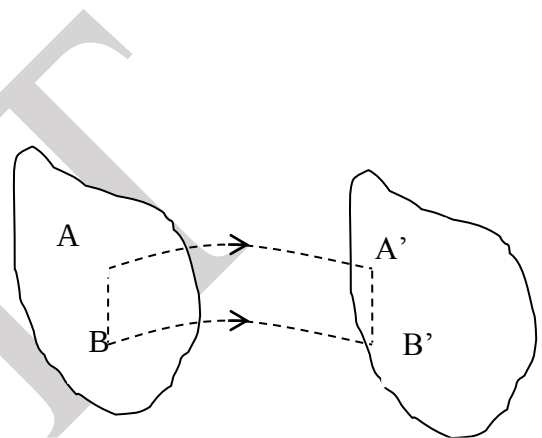
Hình 2-5 Chuyển động tịnh tiến của vật rắn
