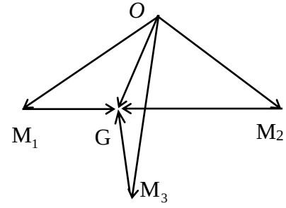
Hình 2-2 Để xác định khối tâm của hệ chất điểm
