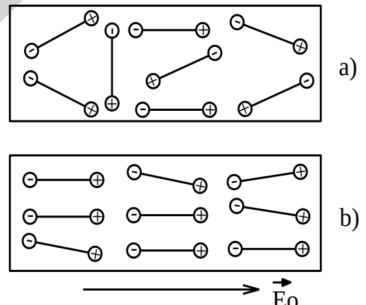
Hình 9-2. Điện môi phân tử tự phân cực
