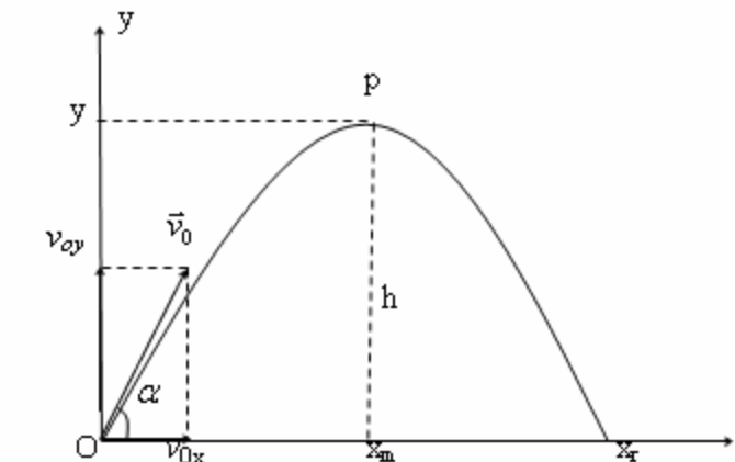
Hình 1-11. Quỹ đạo chuyển động của chất điểm
