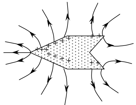
Hình 8-3. Sự phân bố điện tích trên vật dẫn.
