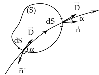
Hình 7-15 Thông lượng gửi qua một mặt kín (S).
