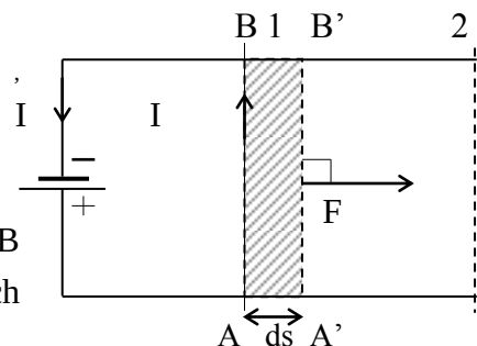
Hình 10-23. Tính công của từ lực
