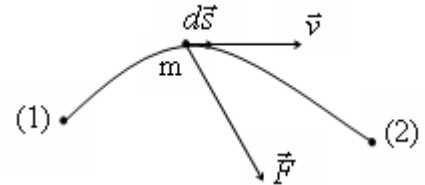
Hình 3-5. Minh họa xác định công của trường lực thế
