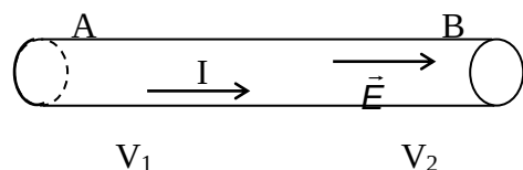
Hình 8-12 Đoạn mạch có dòng điện
