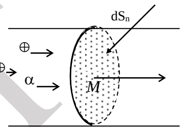
Hình 8-9 Vectơ mật độ dòng
