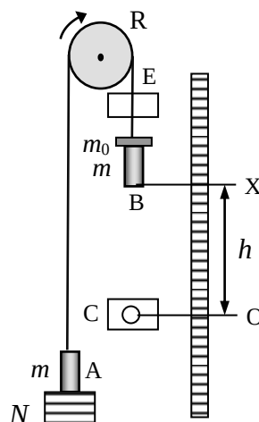
Hình 5: Sơ đồ đo gia tốc, vận tốc trên máy Atwood
