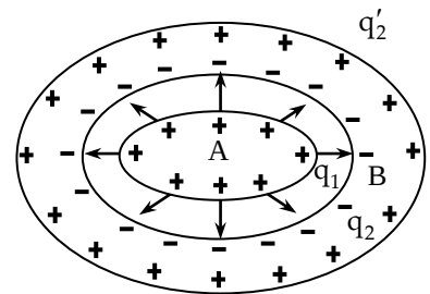
Hình 8- 6. Tụ điện.
