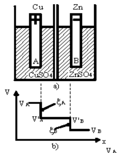
Hình 8-15 Cấu tạo pin Đanien
