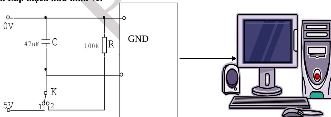
Hình 5: Sơ đồ mạch thí nghiệm về sự phóng điện của tụ điện
