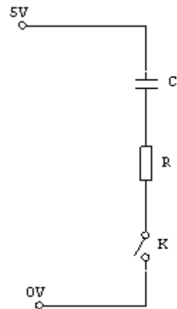
Hình 1: Sơ đồ nguyên lý của quá trình nạp.
