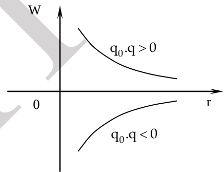
Hình 7-20 Đồ thị thế năng tương tác của hệ hai điện tích điểm.
