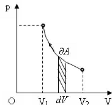
Hình 5-1 Công mà khí nhận được
