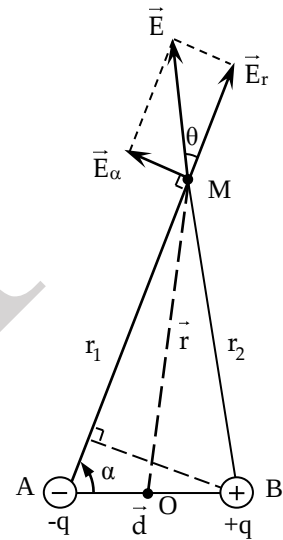
Hình 7-23: Lưỡng cực điện
