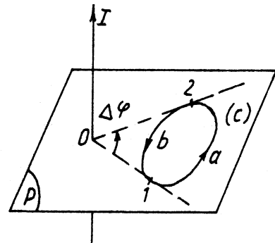
Hình 10-16. Đường cong kín không bao quanh dòng điện
