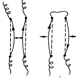
Hình 10-3 Tác dụng giữa hai dòng điện
