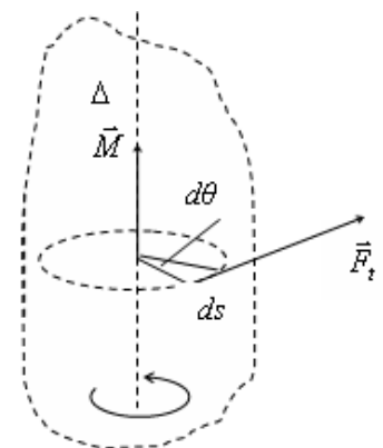
Hình 3-3 Minh họa công của lực trong chuyển động quay
