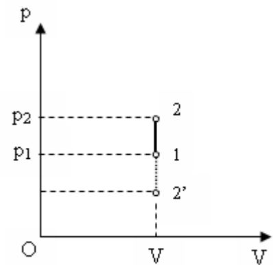
Hình 5-2 Biểu diễn quá trình đẳng tích
