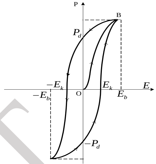
Hình 9 - 6 Chu trình điện trễ
