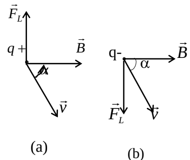
Hình 10-24. Lực Lorentz
