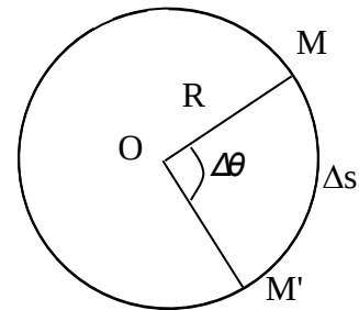
Hình 1-8 Lập công thức vận tốc góc
