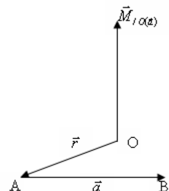
Hình 1-16 Mômen của một véc tơ đối với một điểm
