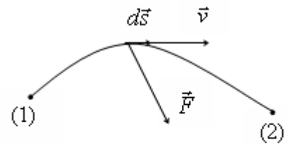
Hình 3-4 Để định nghĩa động năng
