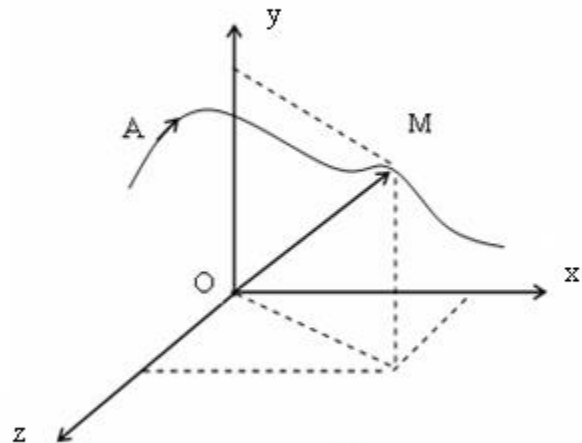
Hình 1- 1 Vị trí của chất điểm
