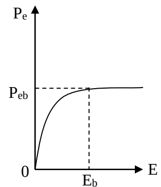
Hình 9-5c Sự phụ thuộc của P_e vào E
