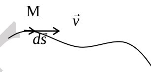
Hình.1-3 Để định nghĩa vector vận tốc
