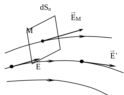
Hình 7-9 Đường sức điện trường.
