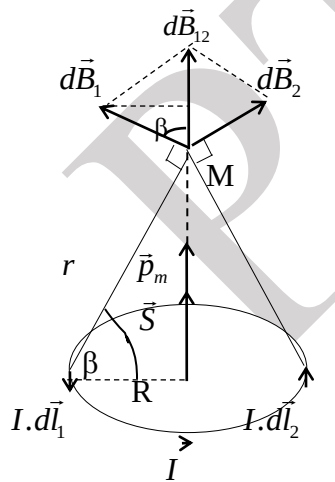
Hình 10-9 Để xác định cảm ứng từ gây bởi dòng điện tròn
