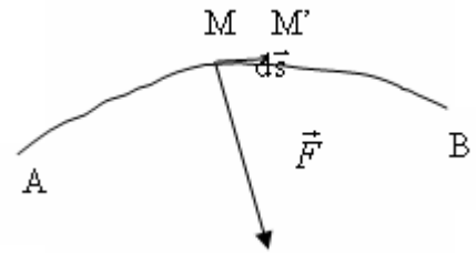
Hình 3-2 Minh họa tính công của lực \vec{F} thay đổi
